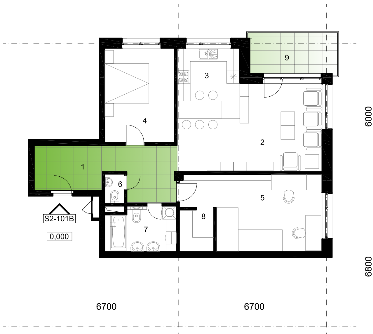
Pôdorys bytu S2-101B M 1:100
