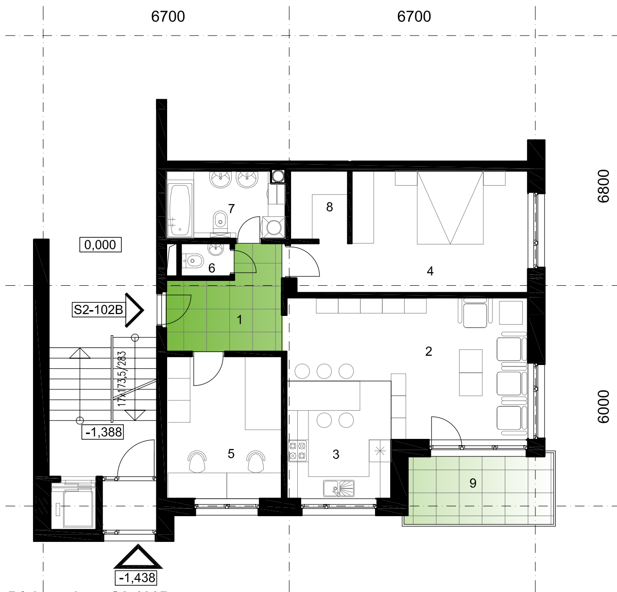
Pôdorys bytu S2-102B M 1:100
