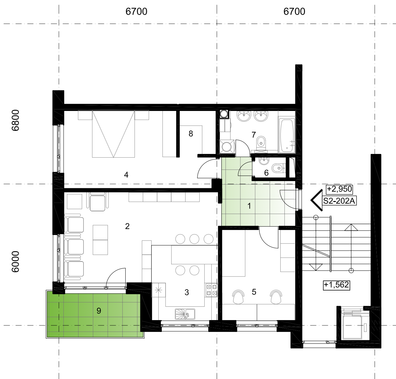
Pôdorys bytu S2-202A M 1:100
