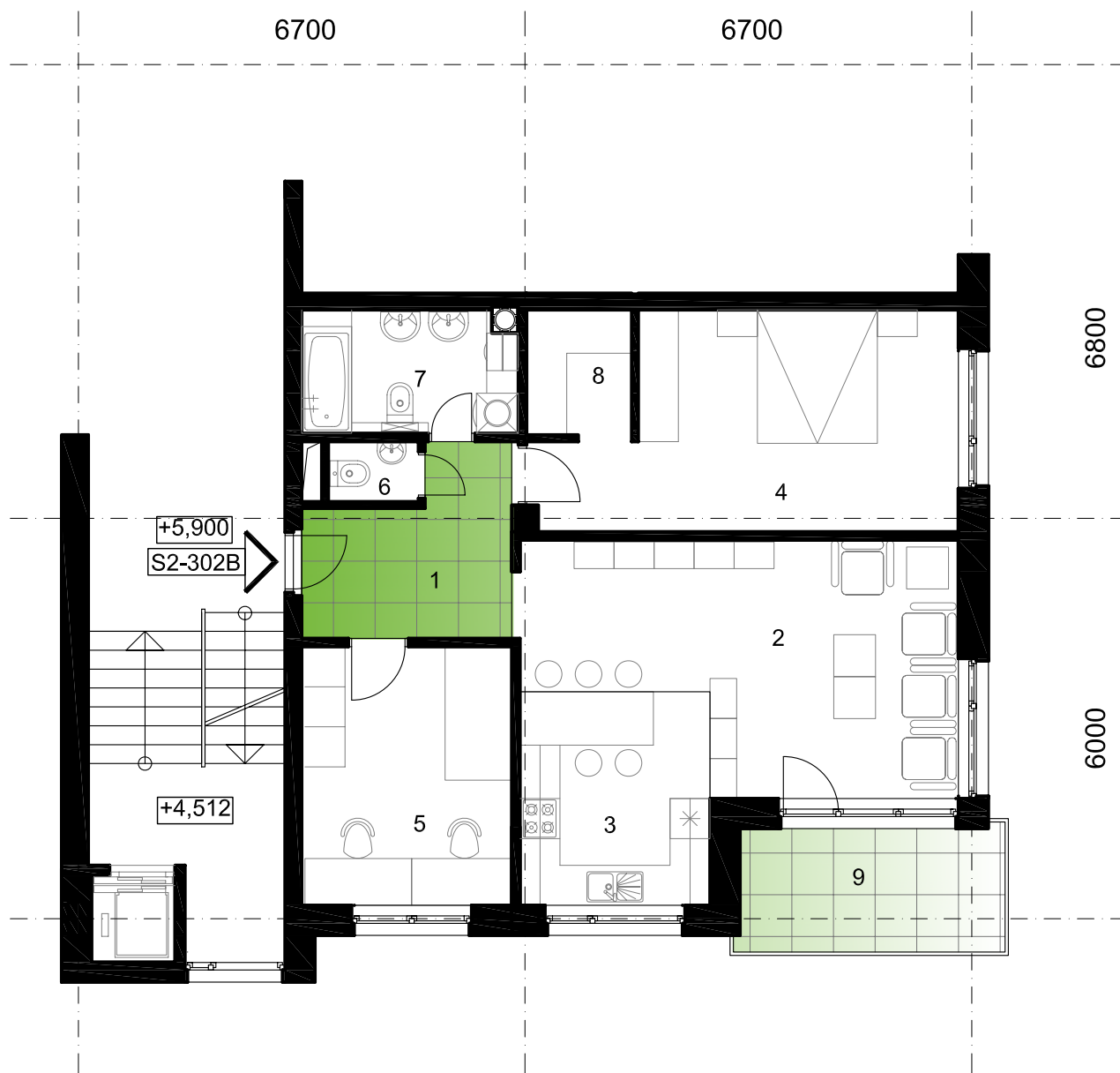
Pôdorys bytu S2-302B M 1:100
